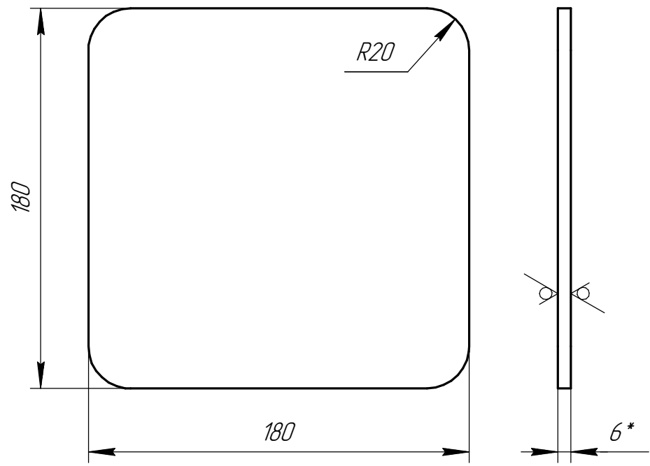
Дет. поз. 2
